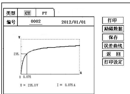
图 5，CT 励磁曲线图
