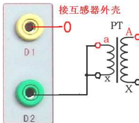
图 21, PT 交流耐压接线图
