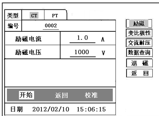
图 3，CT 励磁特性测试界面
