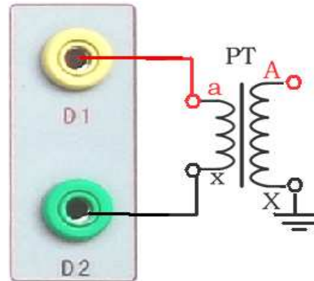
图 16, PT 励磁特性接线图
