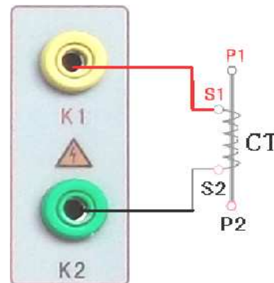
图 4，CT 励磁特性接线图
