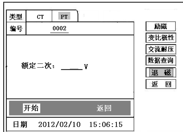
图 17, PT 退磁界面
