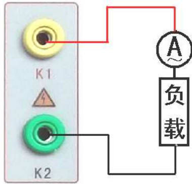
图 27，电流校准接线图
