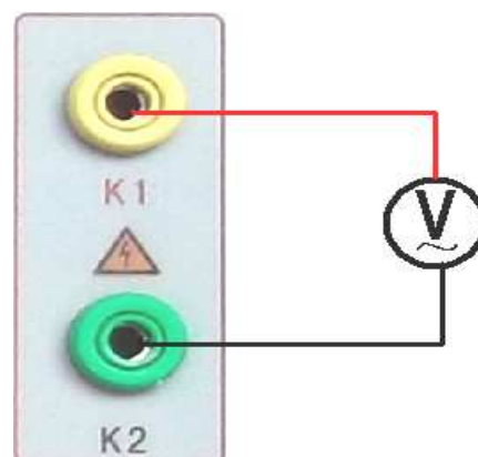
图 26，电压校准接线图
