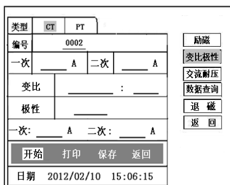
图 11, CT 变比极性测试界面
