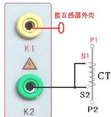
图 14, CT 交流耐压接线图
