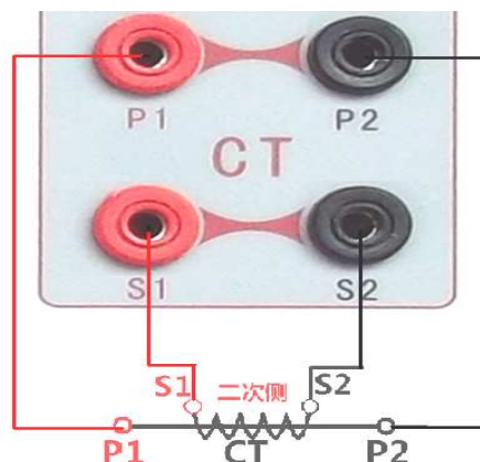
图 12, CT 变比极性接线图
